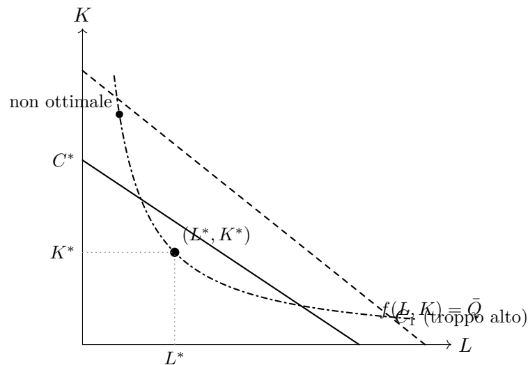
Figura 8.2: Minimizzazione dei costi. L'isocosto C^* è il più basso che raggiunge l'isoquante \bar{Q} . L'isocosto C_1 > C^* interseca l'isoquante (fattibile ma non ottimale: si spende troppo). Il punto di tangenza (L^*, K^*) soddisfa MRTS = w/r .
